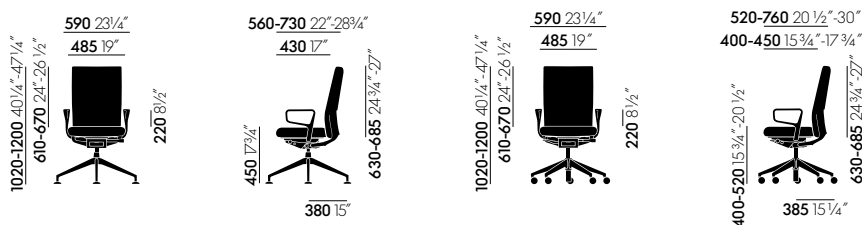
ID Soft L avec accoudoirs fermés fixes
